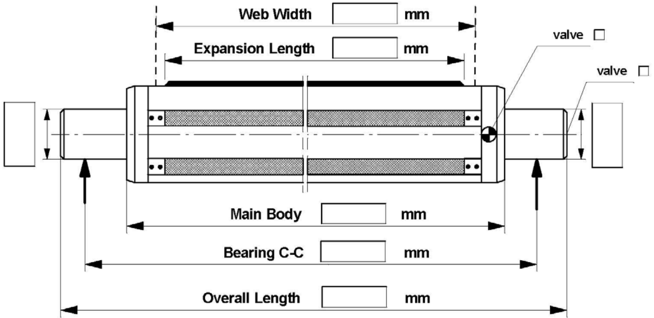
Lug Type Shaft
