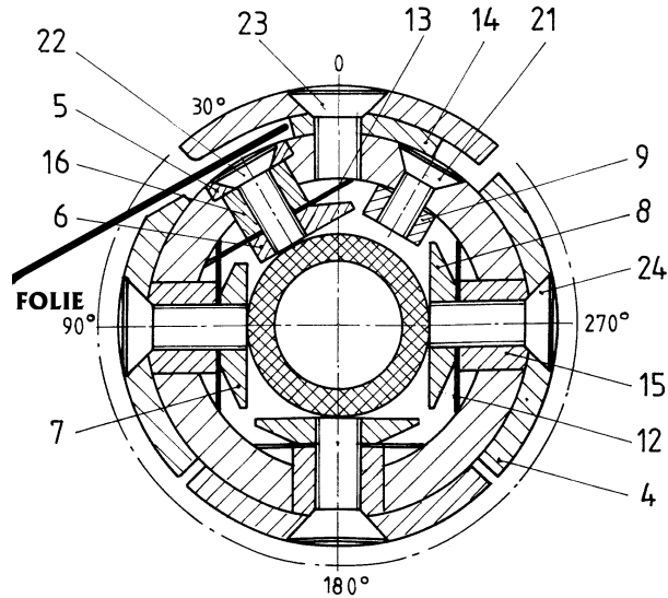
Zeichnung 1: Die Materialbahn, hier mit „Folie“ bezeichnet, wird in der Spalt zwischen feststehender Schale und Greiflamelle eingeschoben.
