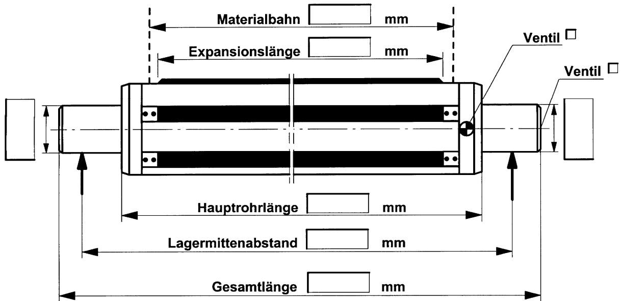
Wellentyp „K“ mit Spann-Keilen
